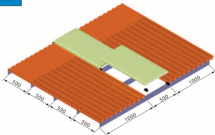
Podlahový systém pro odchov selat s vyhřívanou deskou
